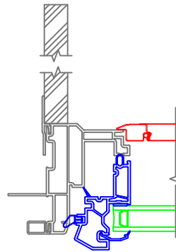
Extension Jamb
